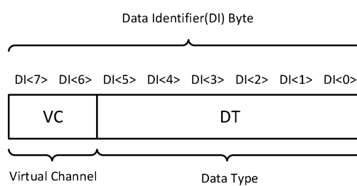
图 1-10 MIPI 数据包 DI 结构
