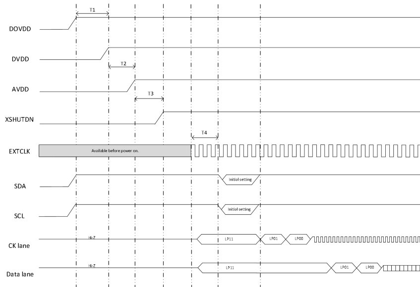
图 1-4 上电时序图
