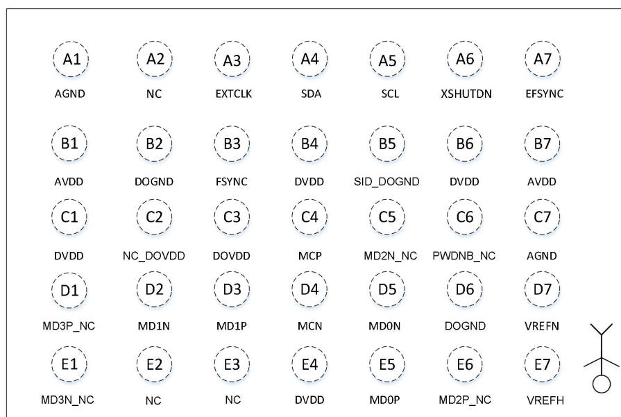
图 1-3 封装引脚图
