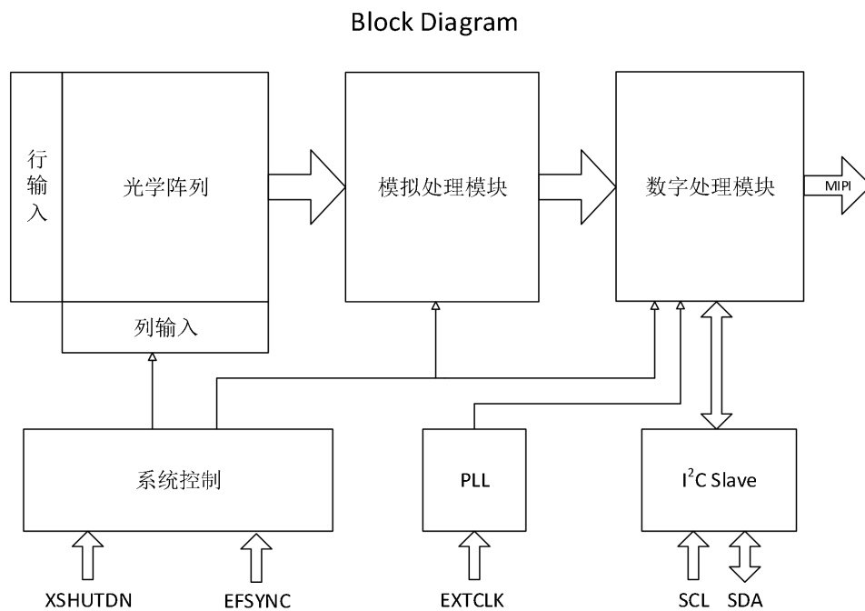
图 1-1 结构图
